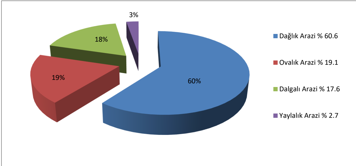
Şekil 3: Topoğrafik yapı
